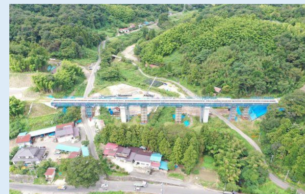
① 第1号橋工事の様子（八島工業(株)付近）
