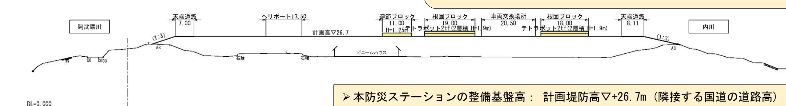
標準断面図
