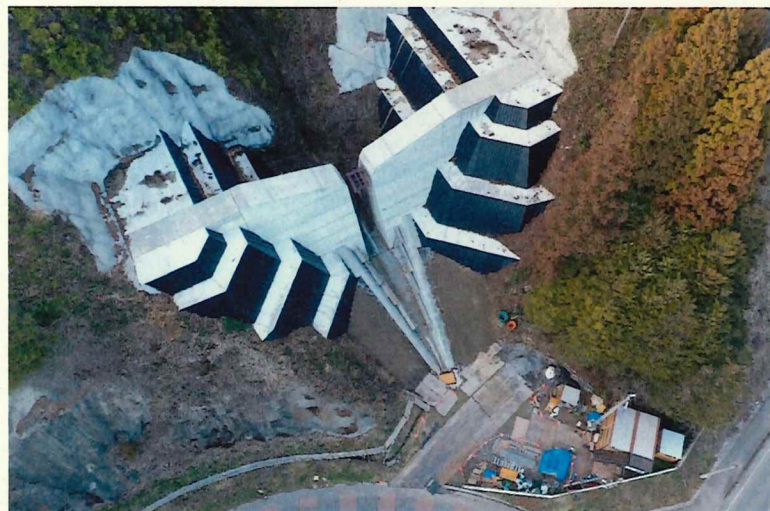
流路工 (擦付護岸工)
