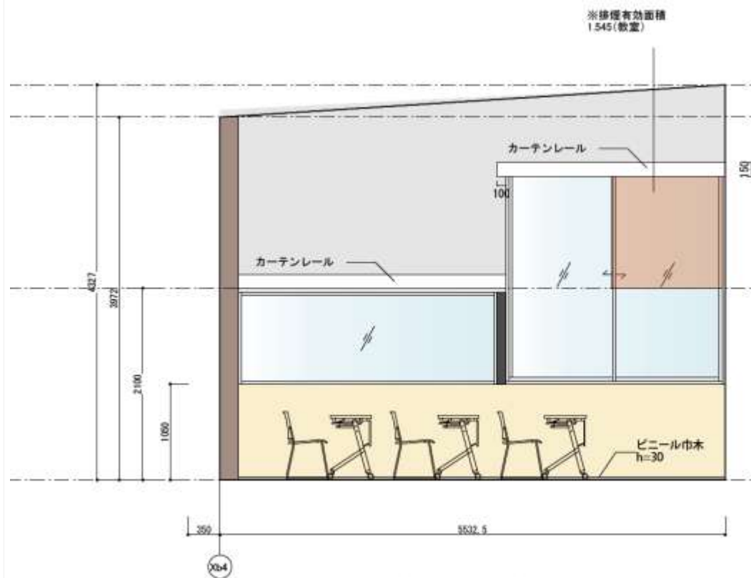
【教室 -A展開】
