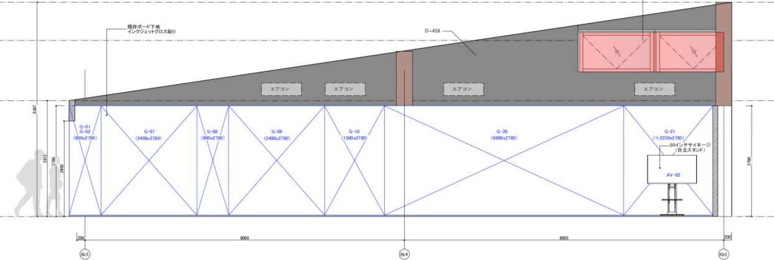
【展示室- B展開】
